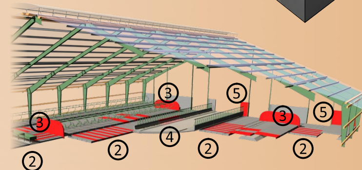
SPODNÍ STAVBA - VARIANTA KEJDOVÉ A PŘERONOVÉ KANÁLY
