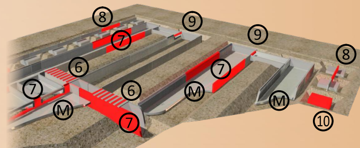
SPODNÍ STAVBA - VARIANTA KEJDOVÉ A PŘERONOVÉ KANÁLY
